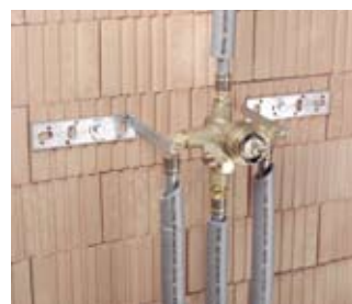
Подключение сантехнических приборов с помощью RAUTITAN.
