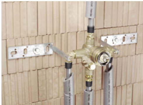
Подключение сантехнических приборов с помощью RAUTITAN
